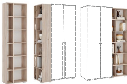
Стеллаж 12 → | Г | ↑ 538|270|2100
