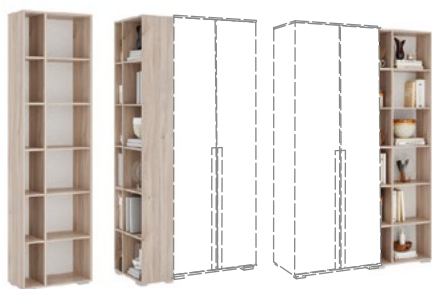
Стеллаж 12 → | 7 | ↑ 538|270|2100
