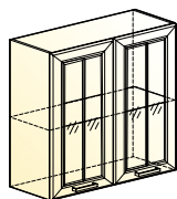
Атланта шкаф навесной (2 двери рамочные) → | 7 | ↑ 800|318|720
