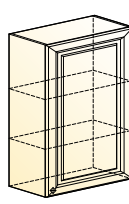
Мишель шкаф навесной (1 дверь глухая) → | 7 | ↑ 600|318|900
