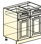
Атланта шкаф рабочий (2 двери 2 ящика) → | 7 | ↑ 800|460|820
