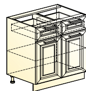
Мишель шкаф рабочий (2 двери 2 ящика) → | 7 | ↑ 800|460|820
