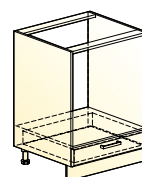
Атланта шкаф рабочий под духовку (1 ящик) → | 7 | ↑ 600|460|820
