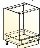
Бавария шкаф рабочий под духовку (1 ящик) → | 1 | 1 | ↑ 600|460|820
