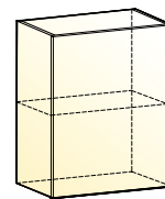
Бостон шкаф навесной (1 дверь глухая) → | 7 | 1 | ↑ 600|318|720
