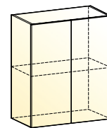
Бостон шкаф навесной (2 двери глухие) → | 7 | 1 | ↑ 600|318|720
