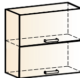
Яна шкаф навесной (2 двери горизонт.) → | 7 | 1 | ↑ 800|318|720
