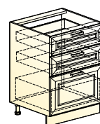
Атланта шкаф рабочий (3 ящика) → | 7 | ↑ 600|460|820
