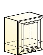
Атланта шкаф навесной под вытяжку (1 дверь глухая) → | 7 | ↑ 600|318|566
