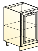
Атланта шкаф рабочий (1 дверь) → | 7 | ↑ 500|460|820
