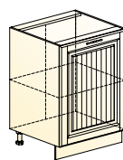
Бавария шкаф рабочий (1 дверь) → | 1 | 1 | ↑ 600|460|820
