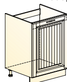
Бавария шкаф рабочий под мойку (1 дверь) → | 1 | 1 | ↑ 600|456|820
