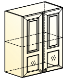
Мишель шкаф навесной (2 двери окошко) → | 7 | 1 ↑ 600|318|720
