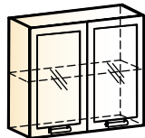
Яна шкаф навесной (2 двери рамочный) → | 7 | 1 | ↑ 800|318|720
