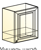
Мишель шкаф навесной под вытяжку (1 дверь глухая) → | 7 | 1 ↑ 600|318|566
