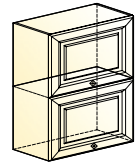
Мишель шкаф навесной (2 двери глухие горизонт.) → | 7 | 1 ↑ 600|318|720
