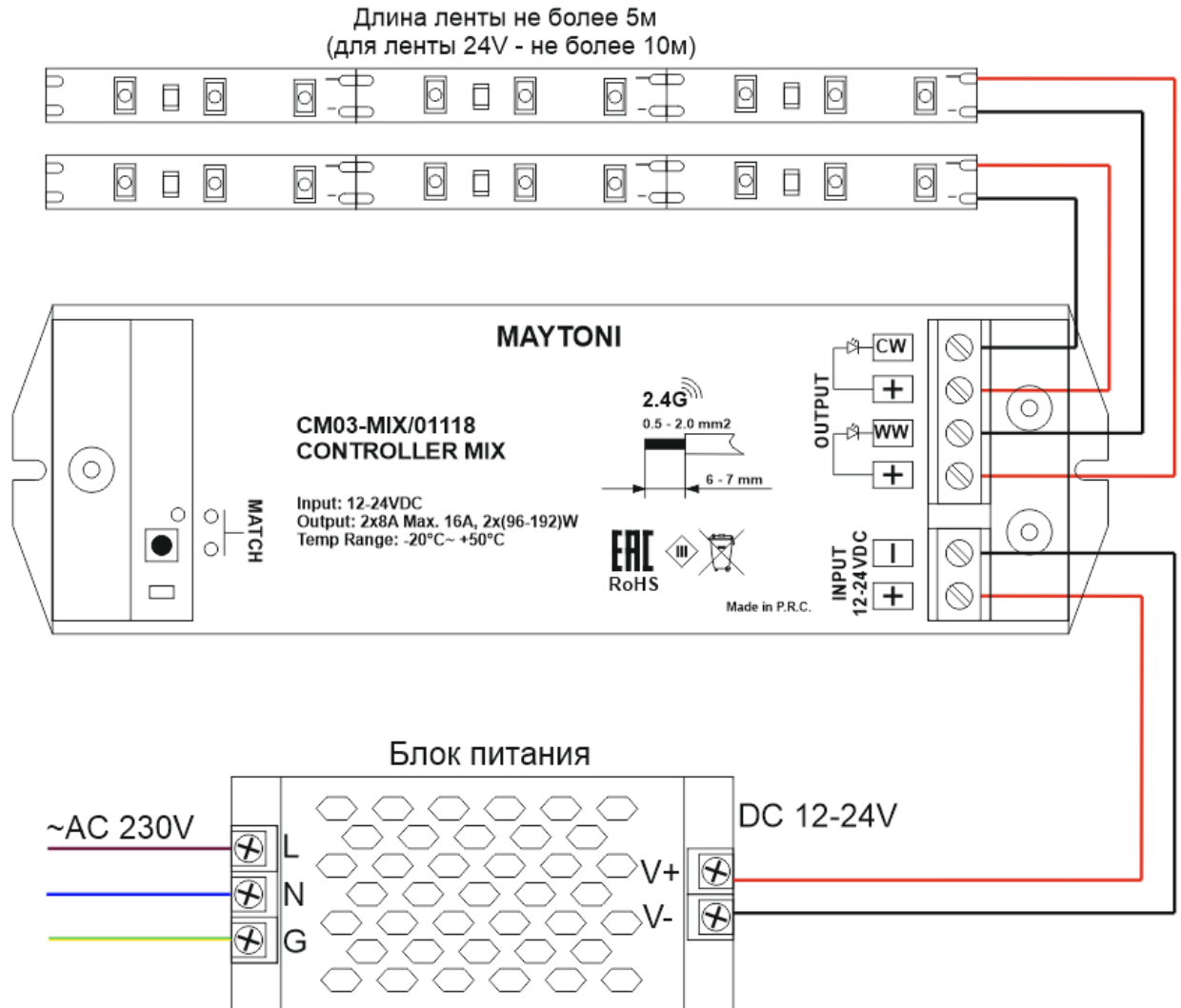
Рис. 2 схема подключения контроллера с использование монохромной ленты
