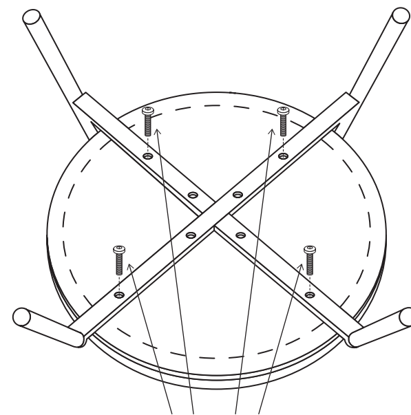
Винты М6х35
